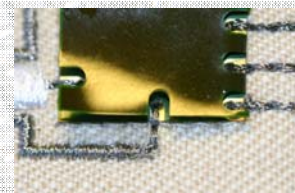
Embroidered Contacts
